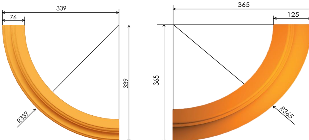
Профіль наружного карнизу №1
